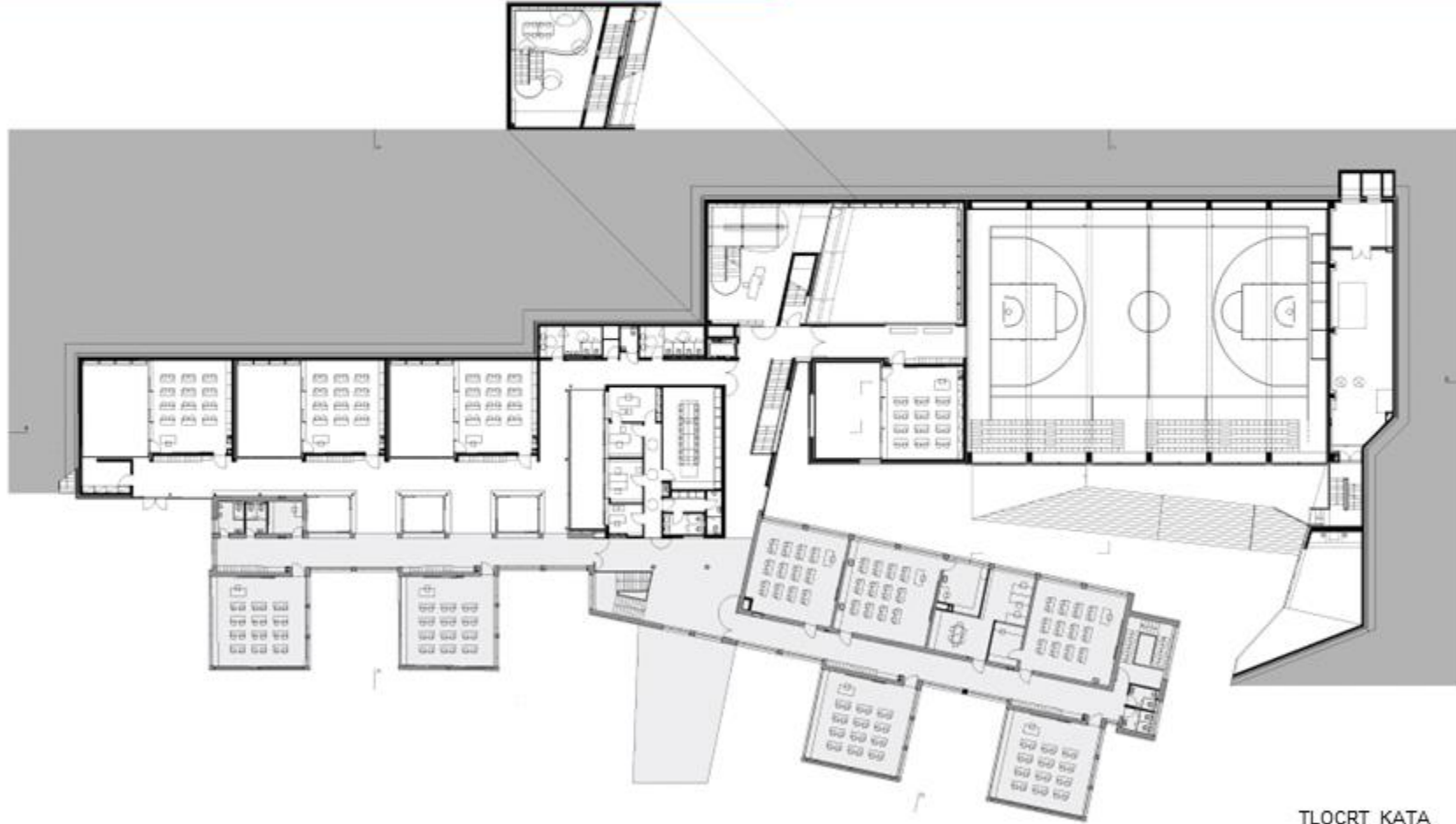
TLOCRT KATA
