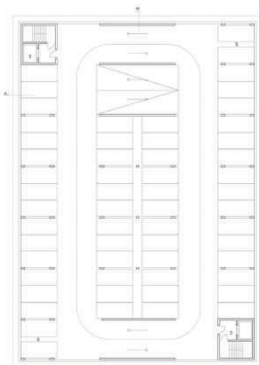
TLOČRT KARAKTERISTIČNE ETAŽE TLOČRT KROVA
