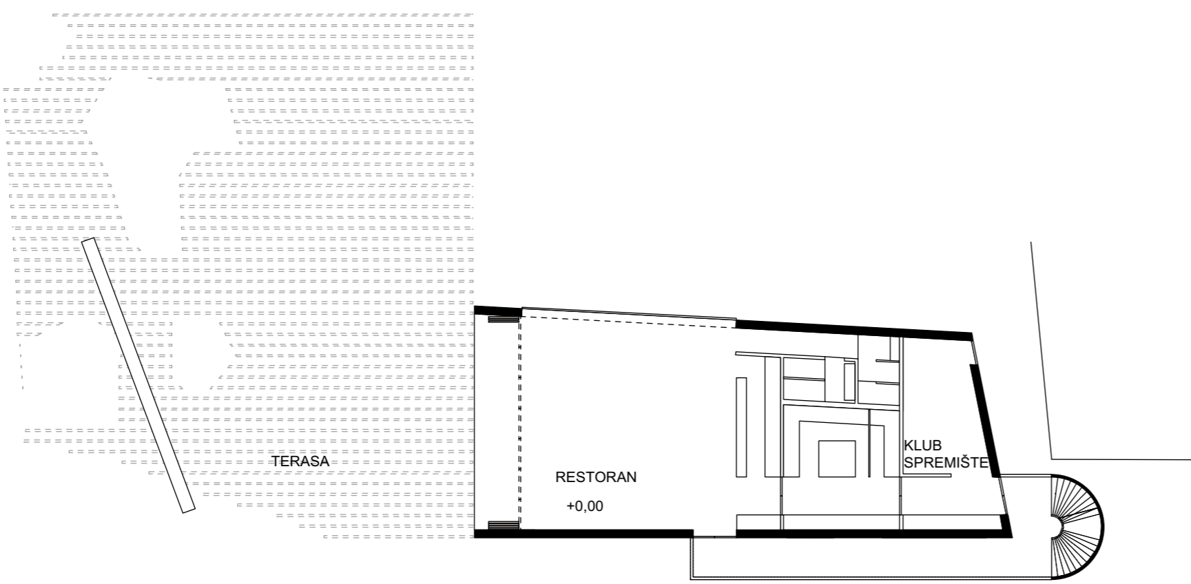
TLOCRT PRIZEMLJE
