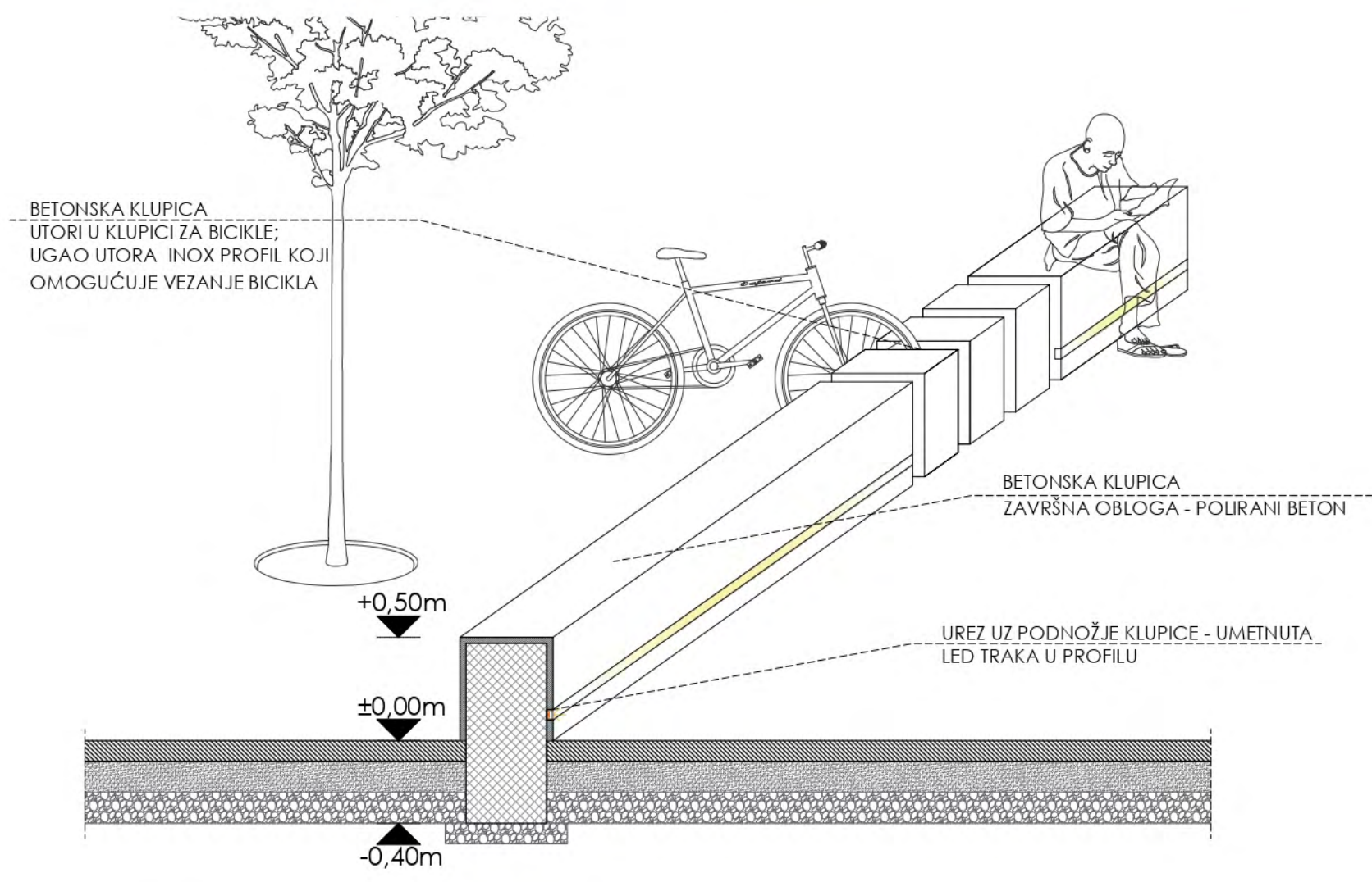
DETALJ / KLUPICA M 1:30
