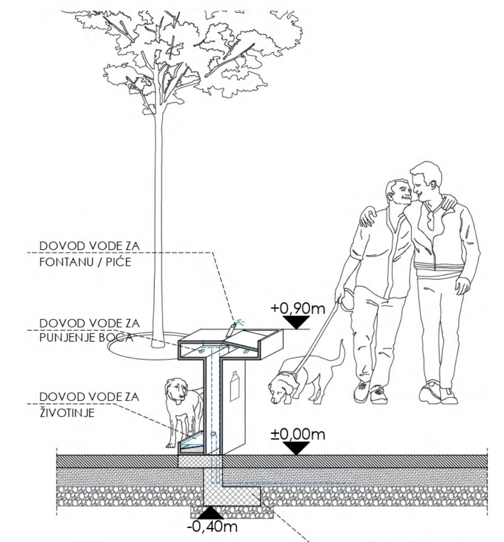
DETALJ / PITKA VODA M 1:30
