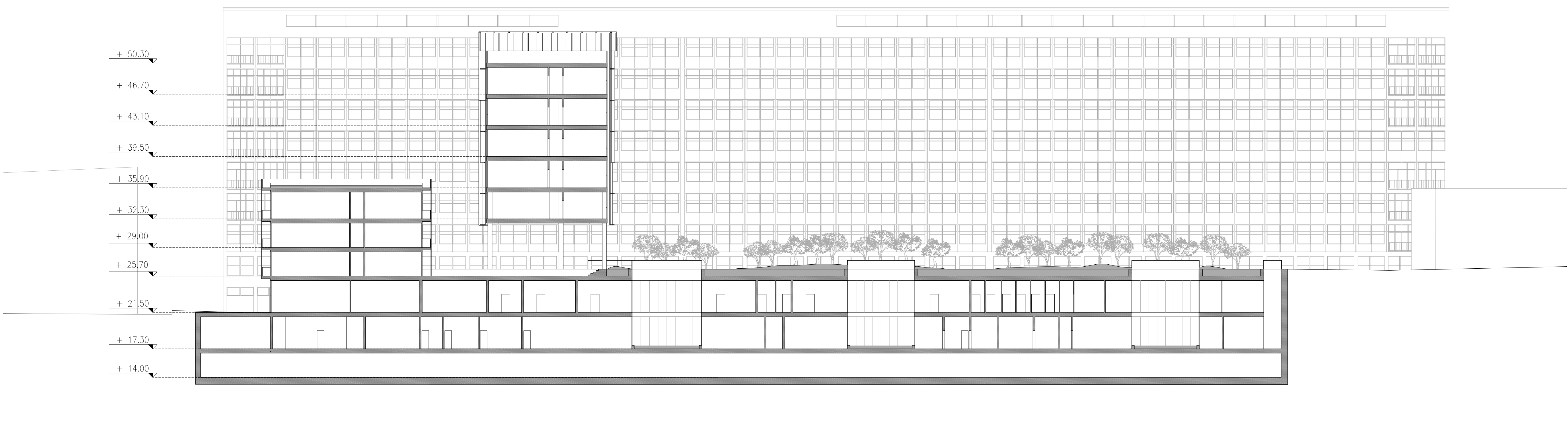
Presjek A-A' 1:250
