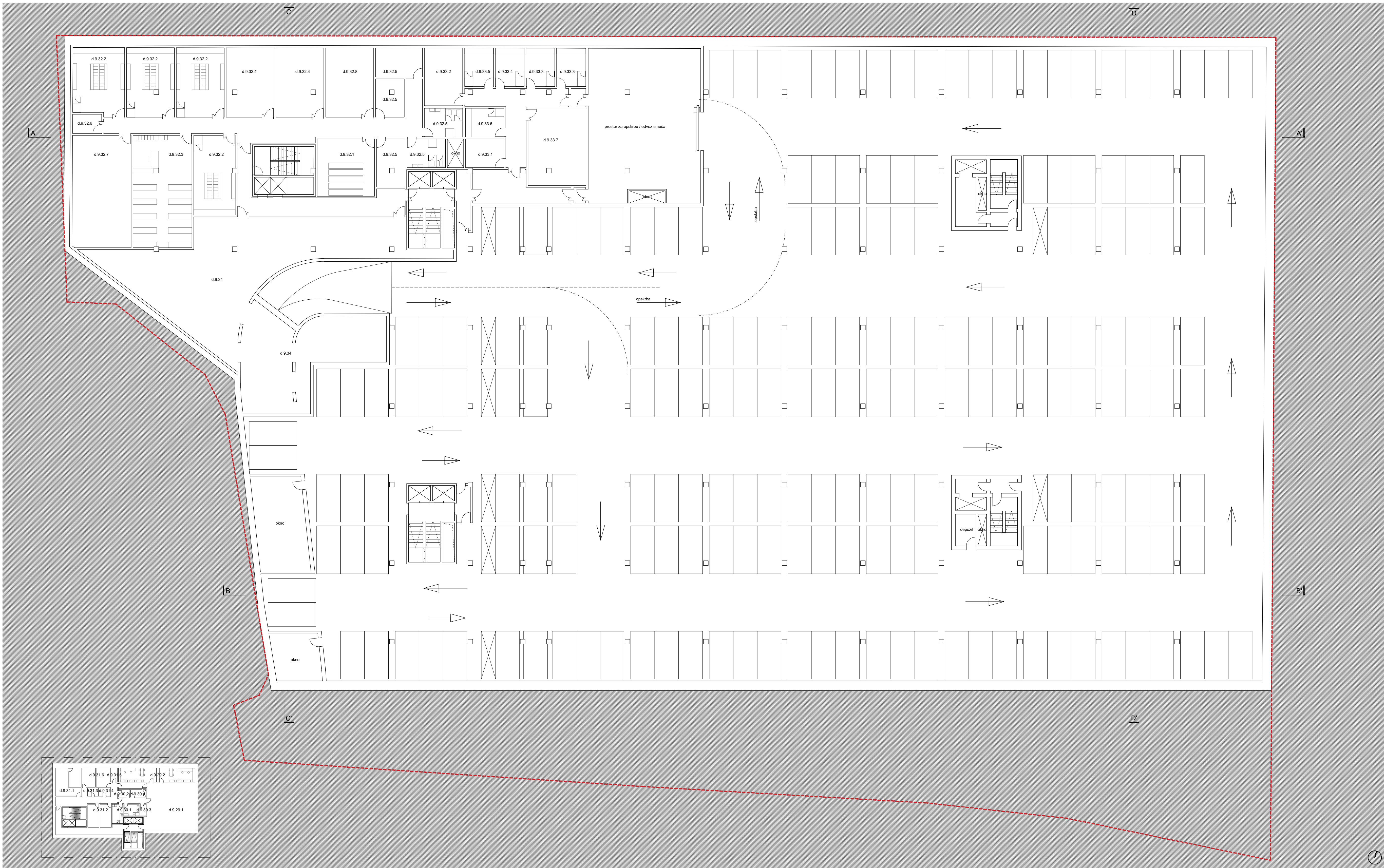
Nivo 10.30 (Vivarium) 1:500
