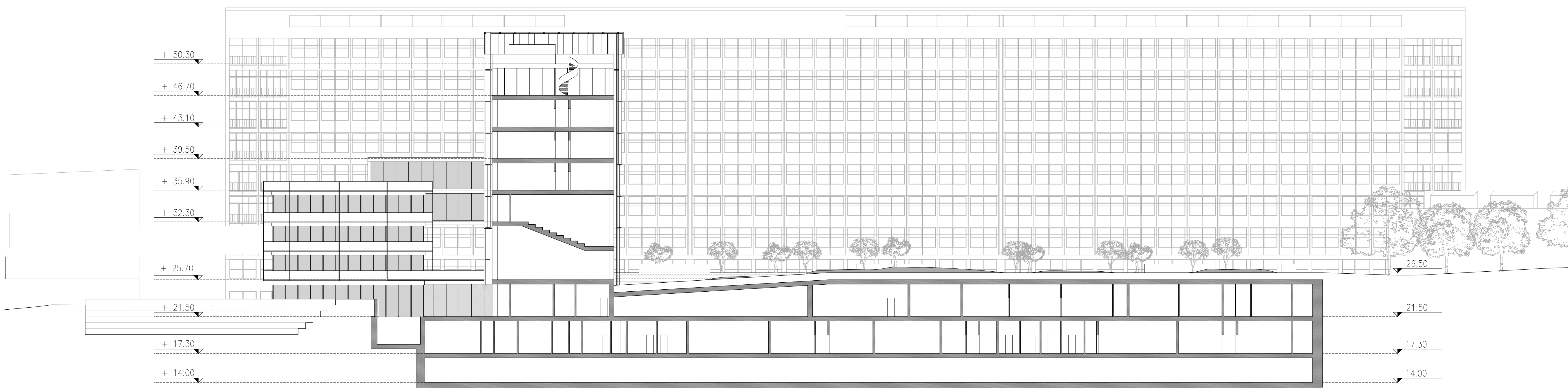
Presjek B-B' 1:250
