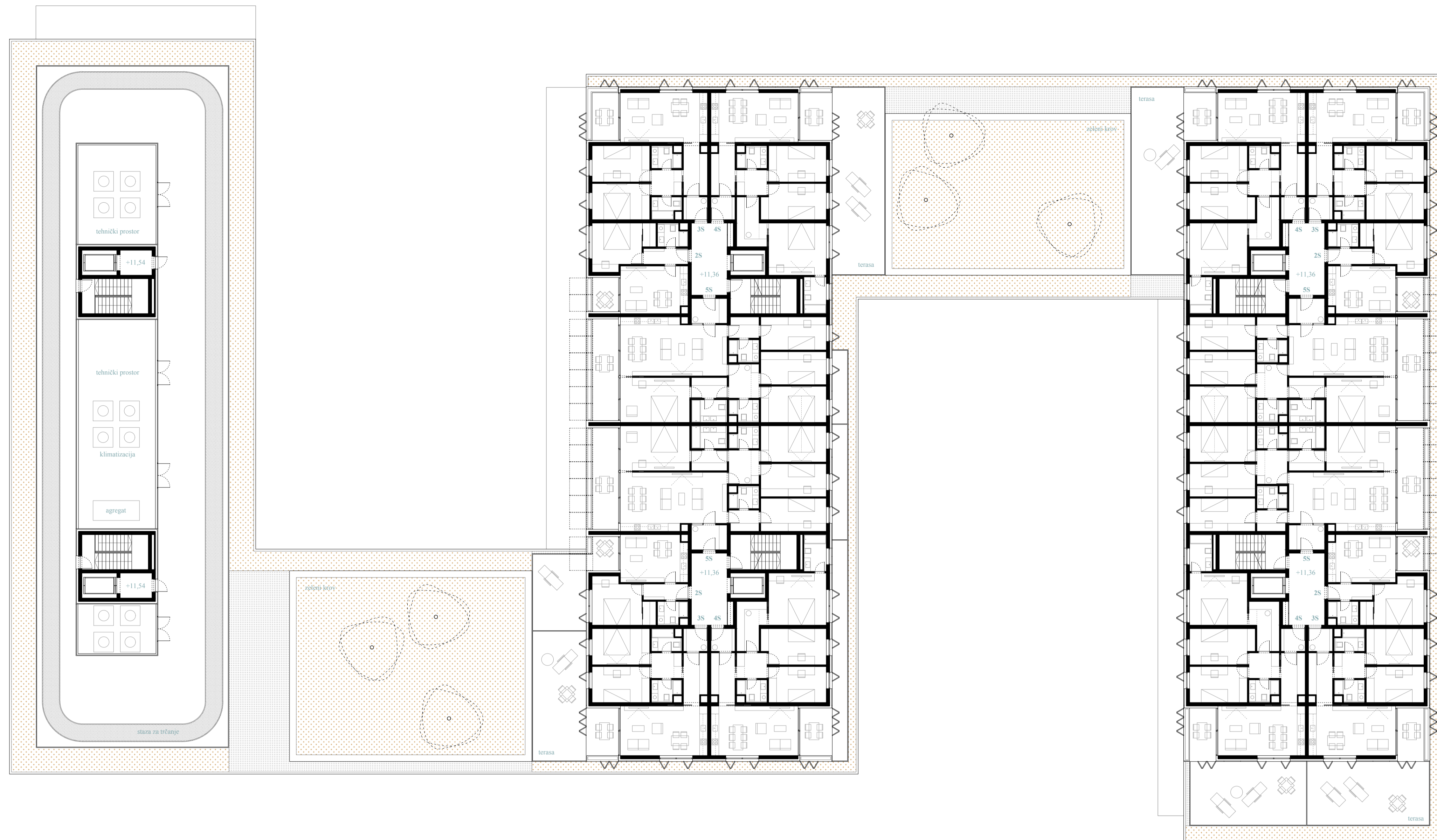
tlocrt krova drugog kata / tlocrt prve stambene etaže: +3 1:200
