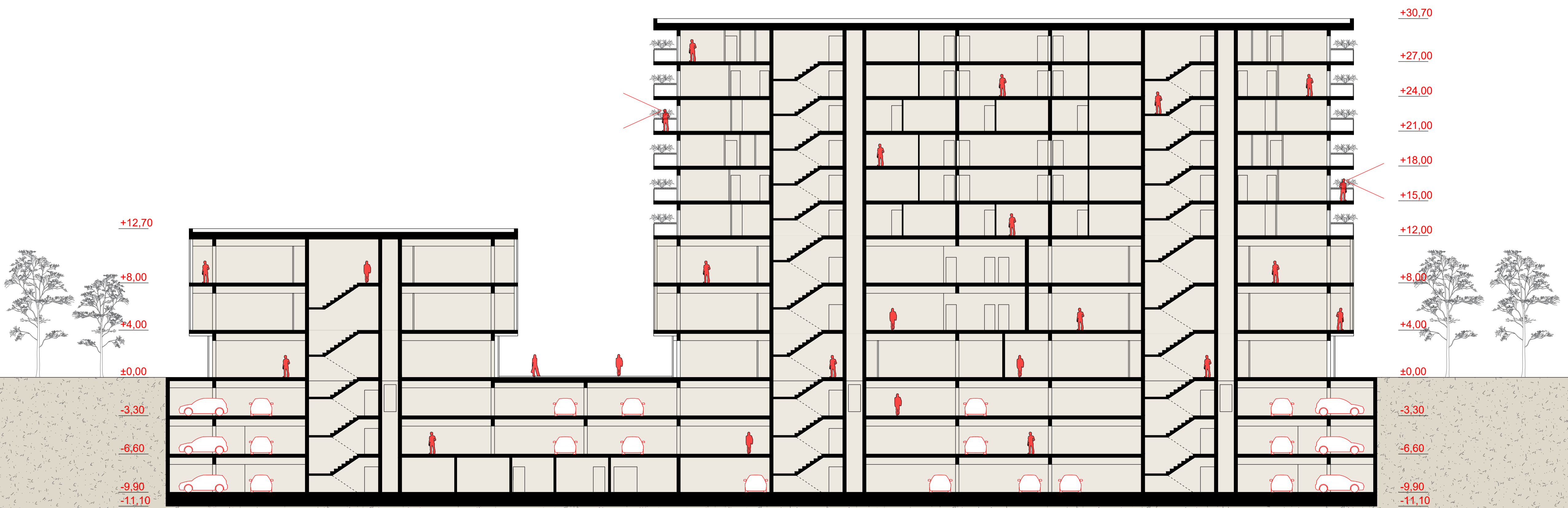
PRESJEK 2-2 M 1:200
