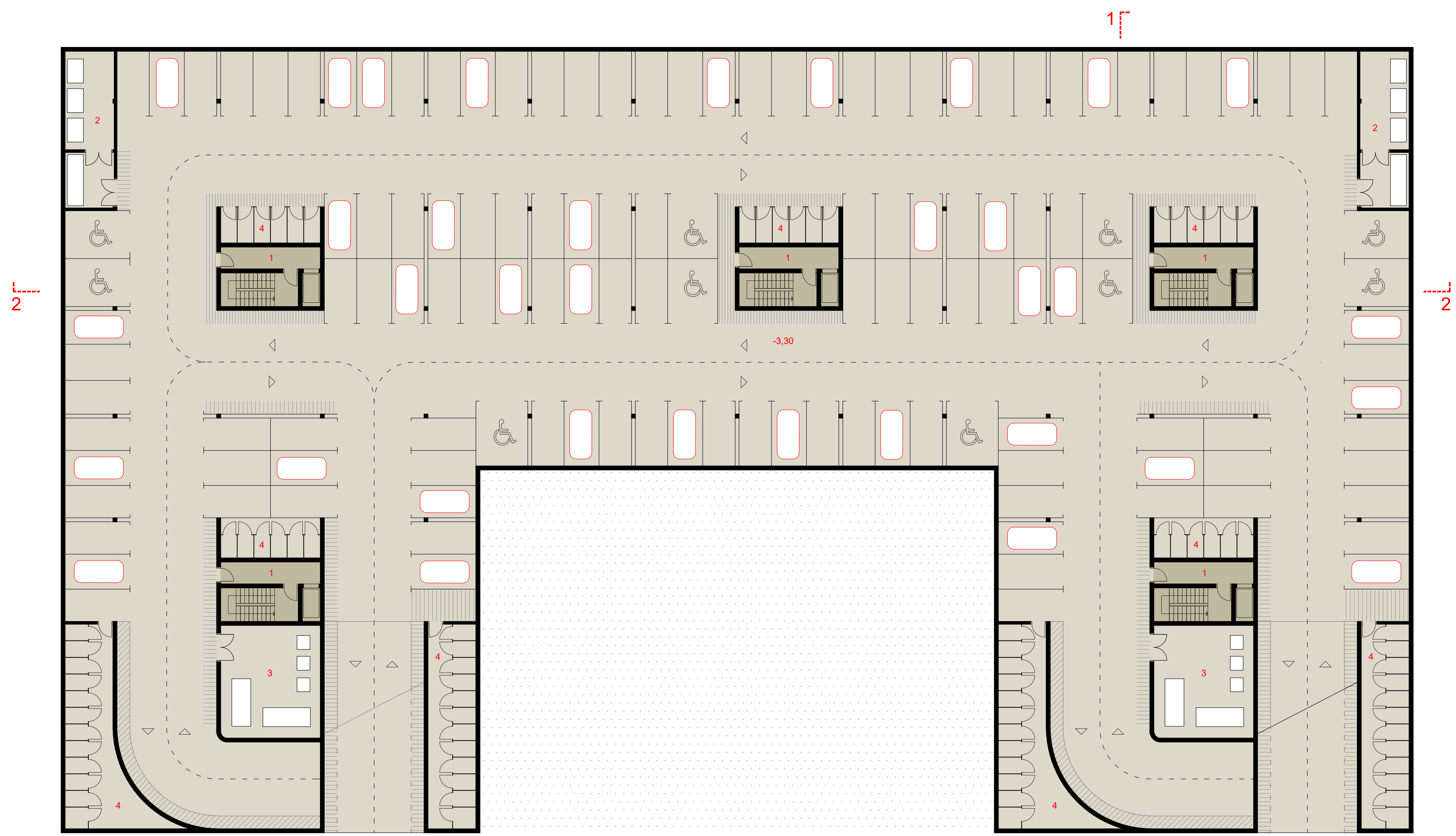
TLOCRT PODZEMNE ETAŽE (-1) M 1:200
