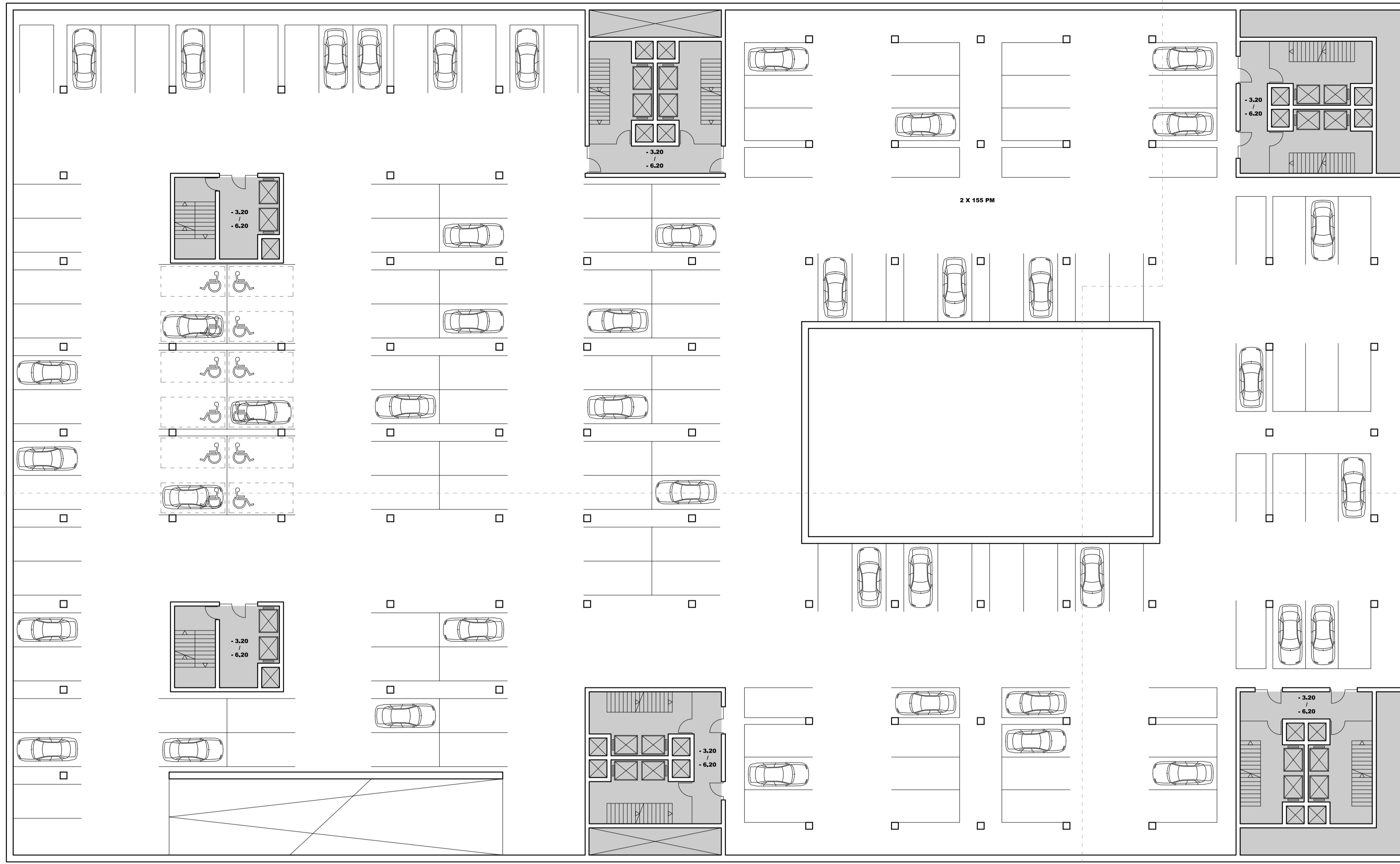
TLOCRT -1 I -2 GARAZE -3,20m / -6,20m M 1:200
