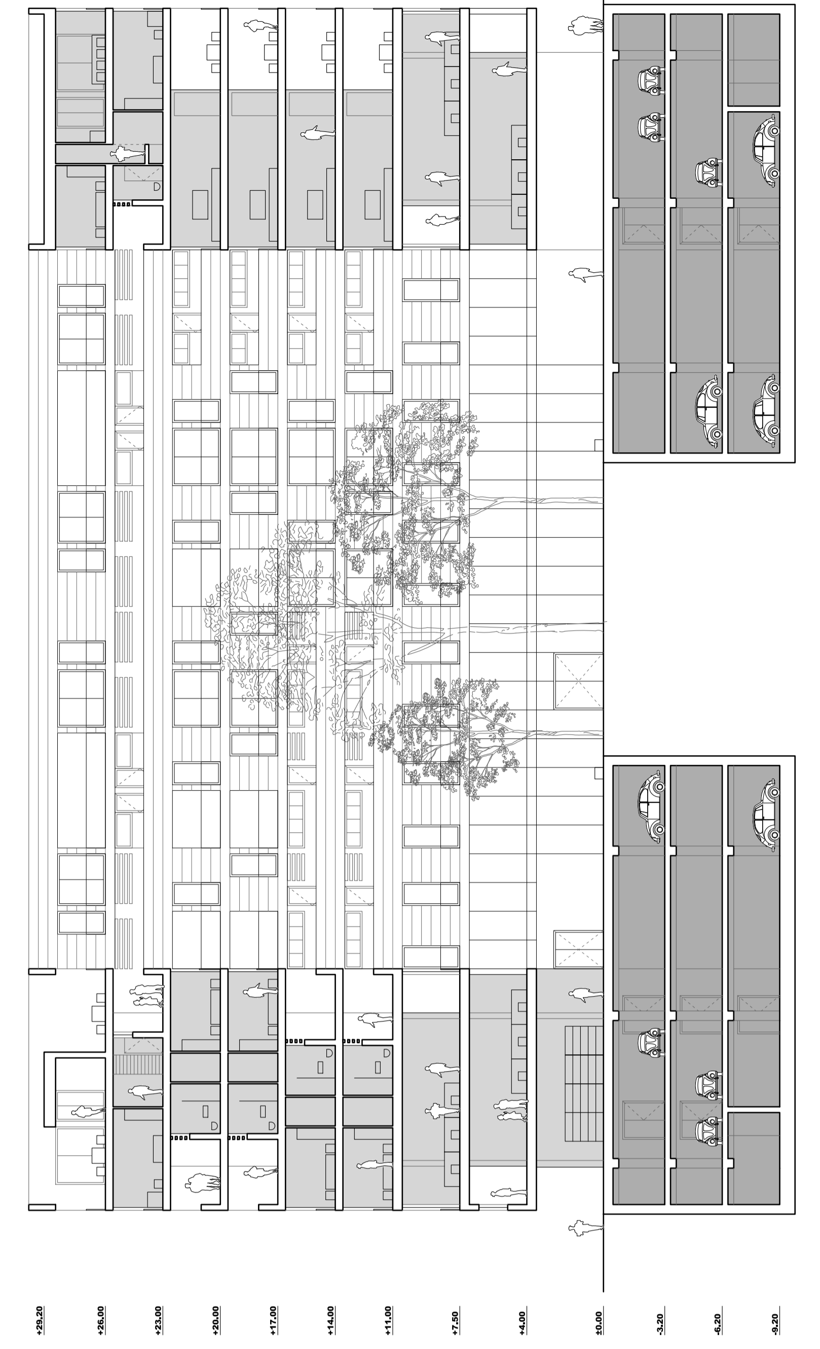
PRESJEK BB M 1:200
