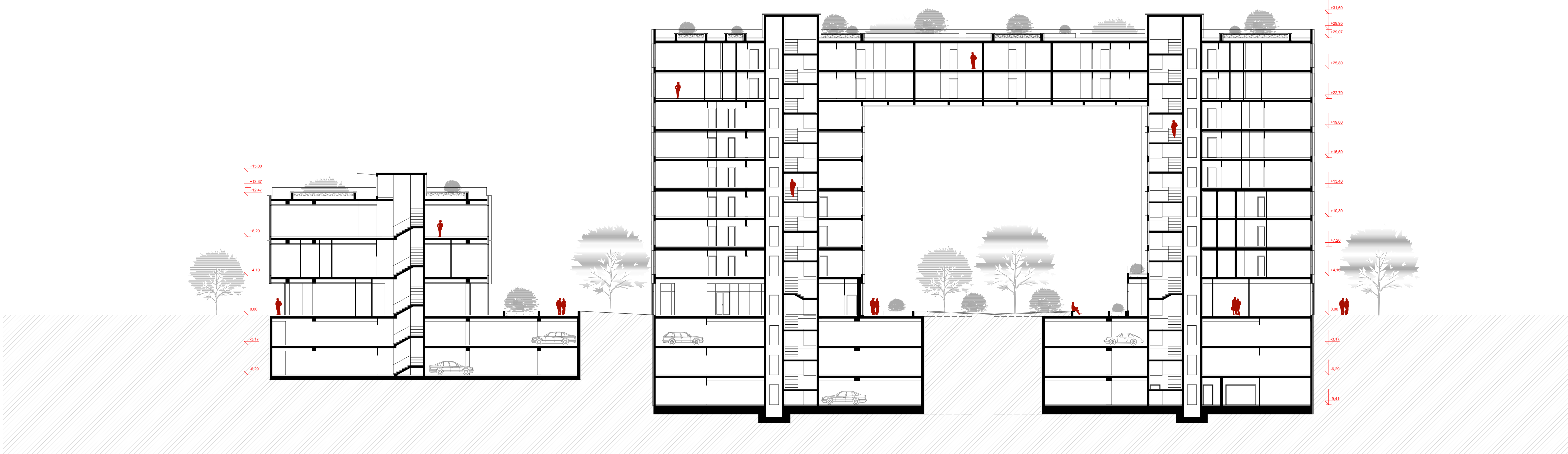
PRESJEK A-A M 1:200 10 15 10
